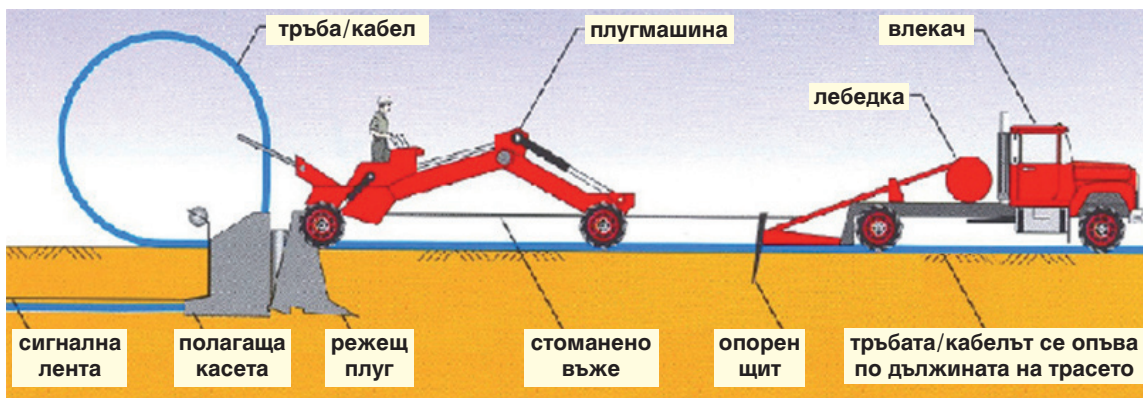
Схема на полагане с плугмашина
